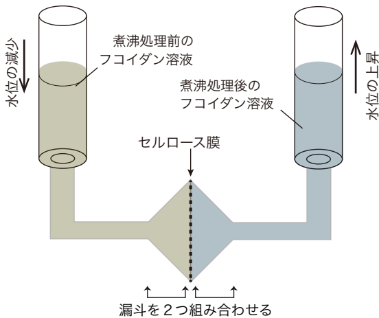
Fig. 2 浸透圧の変化を利用した自作装置
