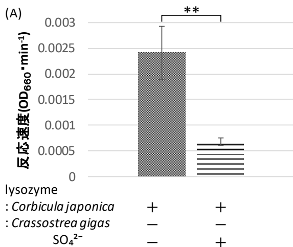
Fig. 5 ヤマトシジミ、マガキの溶菌酵素は硫酸イオンに阻害される ヤマトシジミ ( Corbicula japonica ) 粗酵素液の反応系(A), マガキ ( Crassostrea gigas ) 粗酵素液の反応系(B). **: p < 0.05
