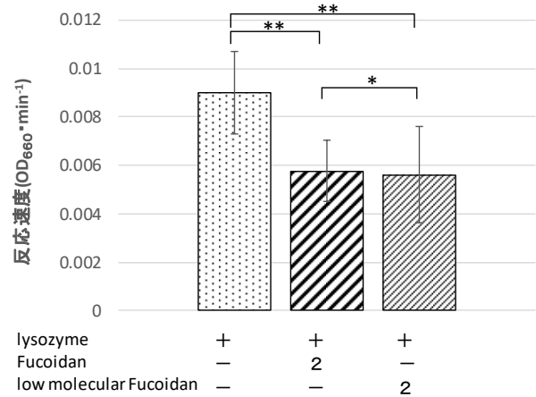
Fig. 3 フコイダンの分子量はリゾチーム阻害に関与しない 基質: E. coli **: p<0.10 *: p>0.10
