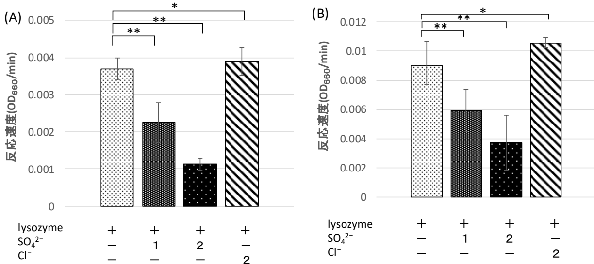
Fig. 1 硫酸イオンはリゾチームを阻害する (A)基質: B. subtilis , (B)基質: E. coli , **: p<0.05 *: p>0.05
