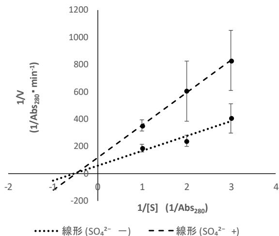
Fig. 4 Lineweaver-Burk plot による阻害様式判定 基質: B. subtilis 乾燥菌体 すべての基質濃度において SO_4^{2-}+ と SO_4^{2-}- が p < 0.05
