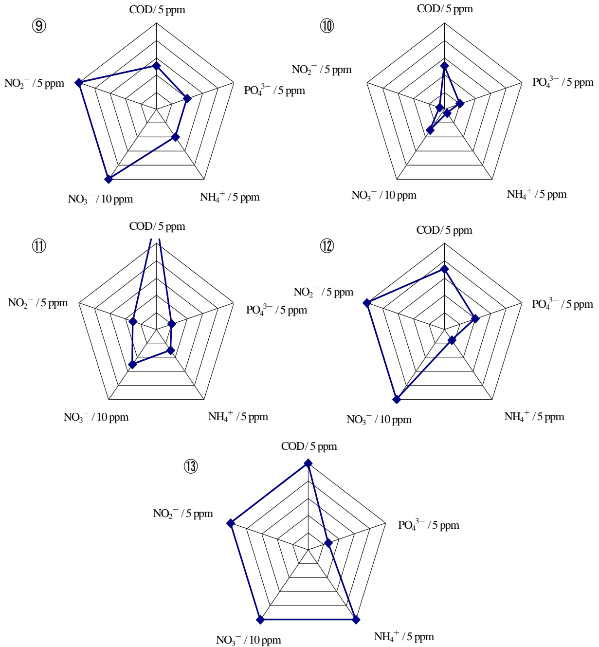
図3 13ポイントのCOD, NO 2 - , NO 3 - , PO 4 3- , NH 4 + 濃度のペンタダイアグラム
