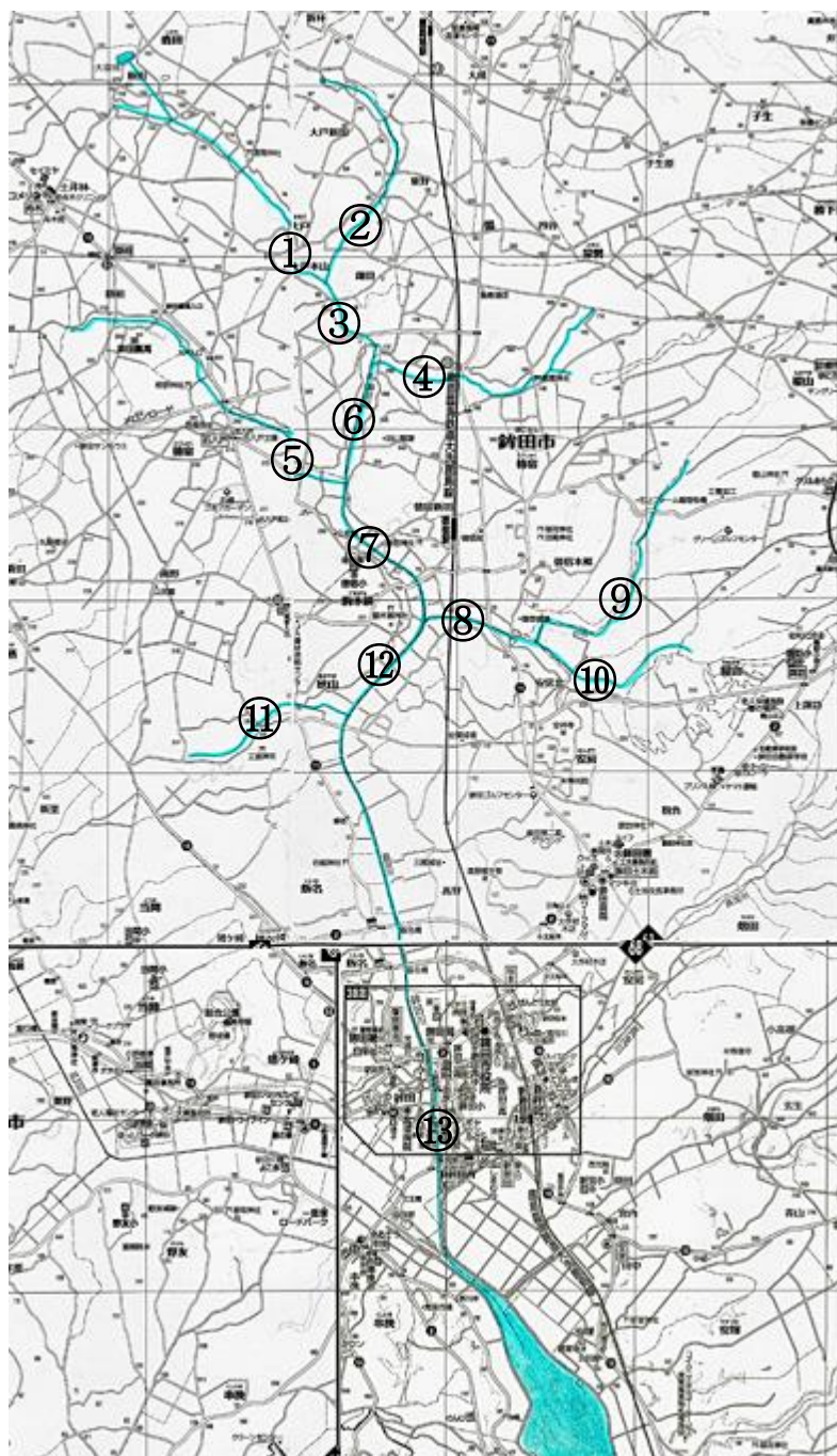
図2 鉾田川全域地図と調査ポイント
