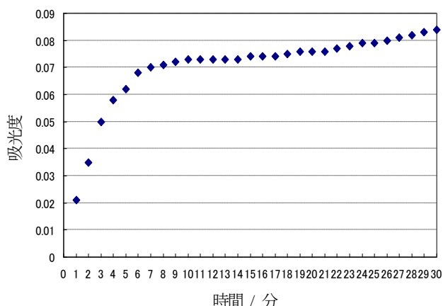
図10 NO 3 - 濃度が3ppmのパックテスト試薬溶液における吸光度の時間変化
