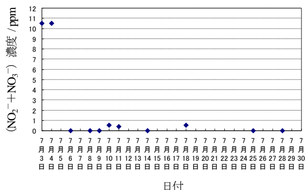
図4 水槽Aの( \text{NO}_2^- + \text{NO}_3^- )濃度の変化
