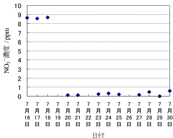
図 15 窒素置換された水槽における \text{NO}_3^- 濃度の変化
