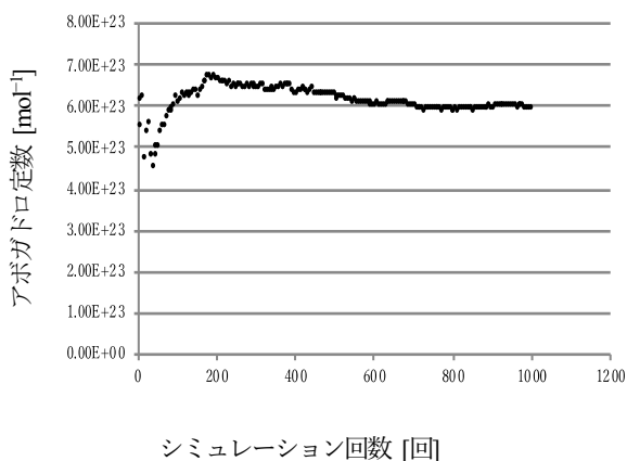
Fig.1 : シミュレーション回数とアボガドロ定数
