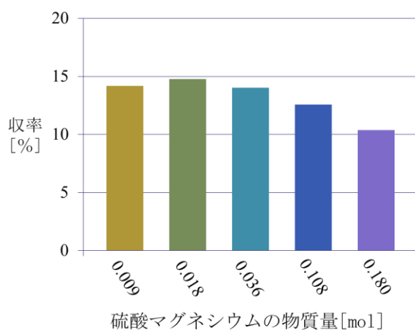
図6 酸触媒を酢酸、脱水剤を硫酸マグネシウムに固定し、脱水剤の物質質量を変化させたときのその収率の変化
