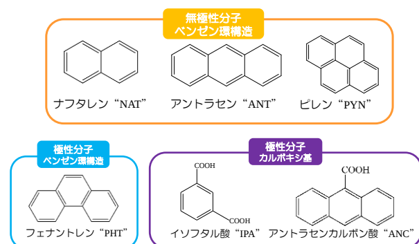
図1 本実験で用いた物質の分子構造
