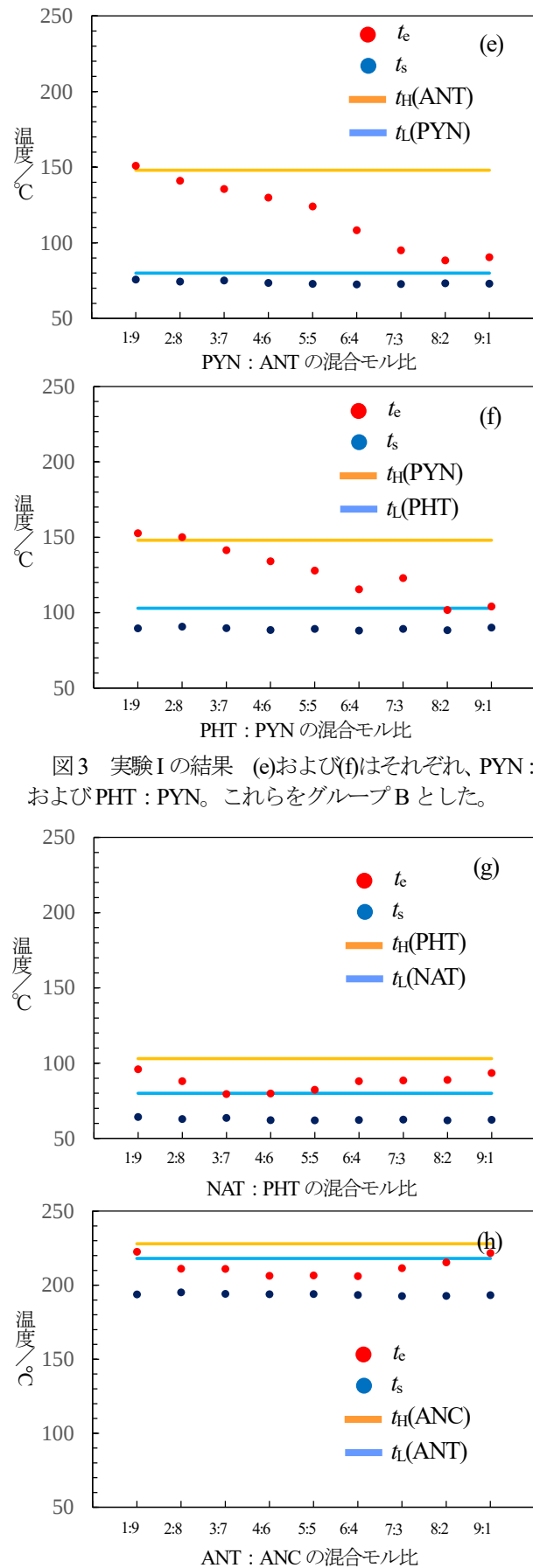
図4 実験Iの結果 (g)および(h)はそれぞれ、NAT : PHT およびANTC : ANC。これらをグループCとした。
